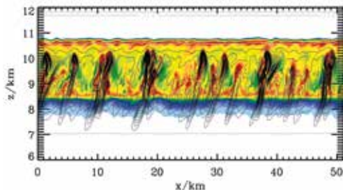
Computersimulation von konvektiven Zellen in Eiswolken
